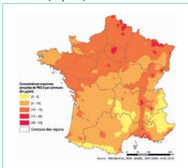
Concentrations moyennes annuelles de PM 2,5 en France continentale (2007-2008)
